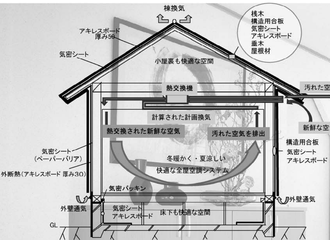
高断熱・高気密+計画換気のイメージ図
